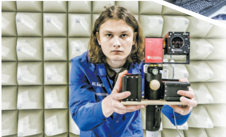
Малады спецыяліст, тэхнік выпрабавальнага цэнтра БелДІСС Андрэй РАМАНАЎ наладжвае абсталяванне для відэафіксацыі выпрабаванняў прадукцыі па электрамагнітнай сумяшчальнасці.
