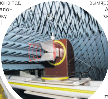
Нацыянальны эталон адзінкі шчыльнасці патоку нейтронаў і электрамагнітнага поля.
